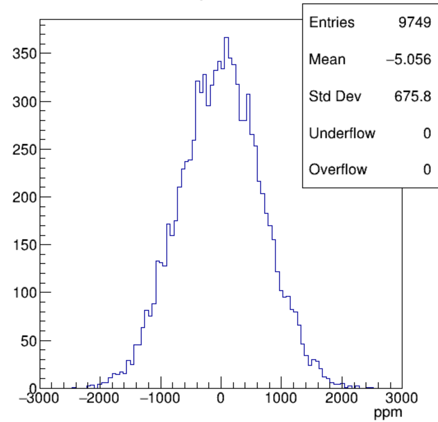
asym_usl
