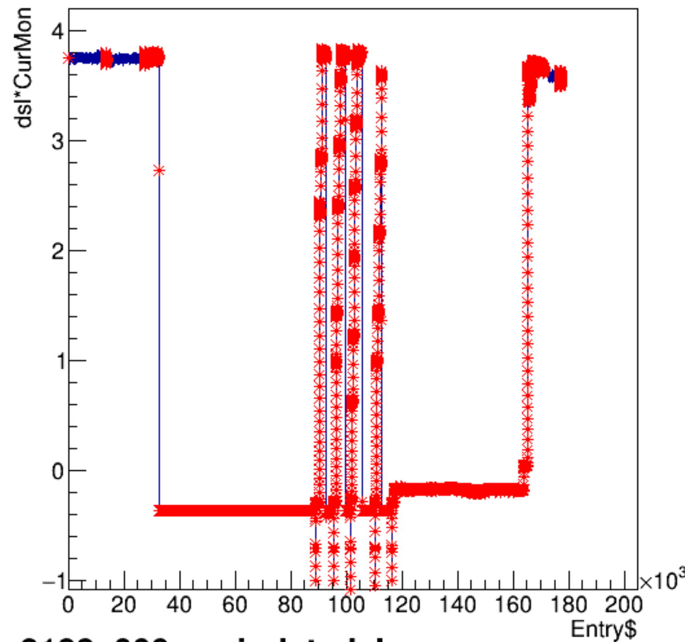
dsl*CurMon:Entry$
