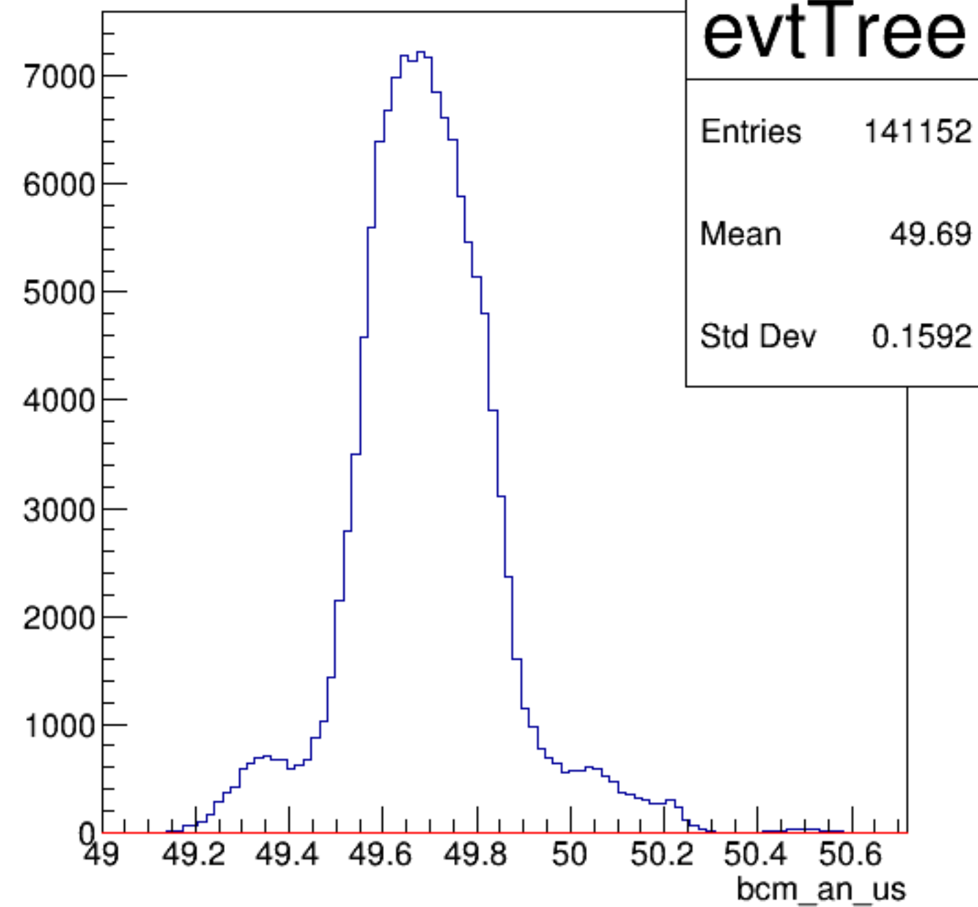
bcm_an_us {ErrorFlag==0}
