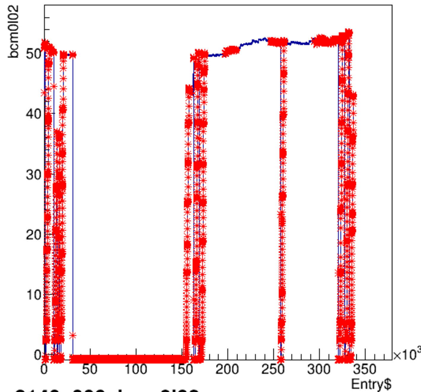
bcm0l02:Entry$
