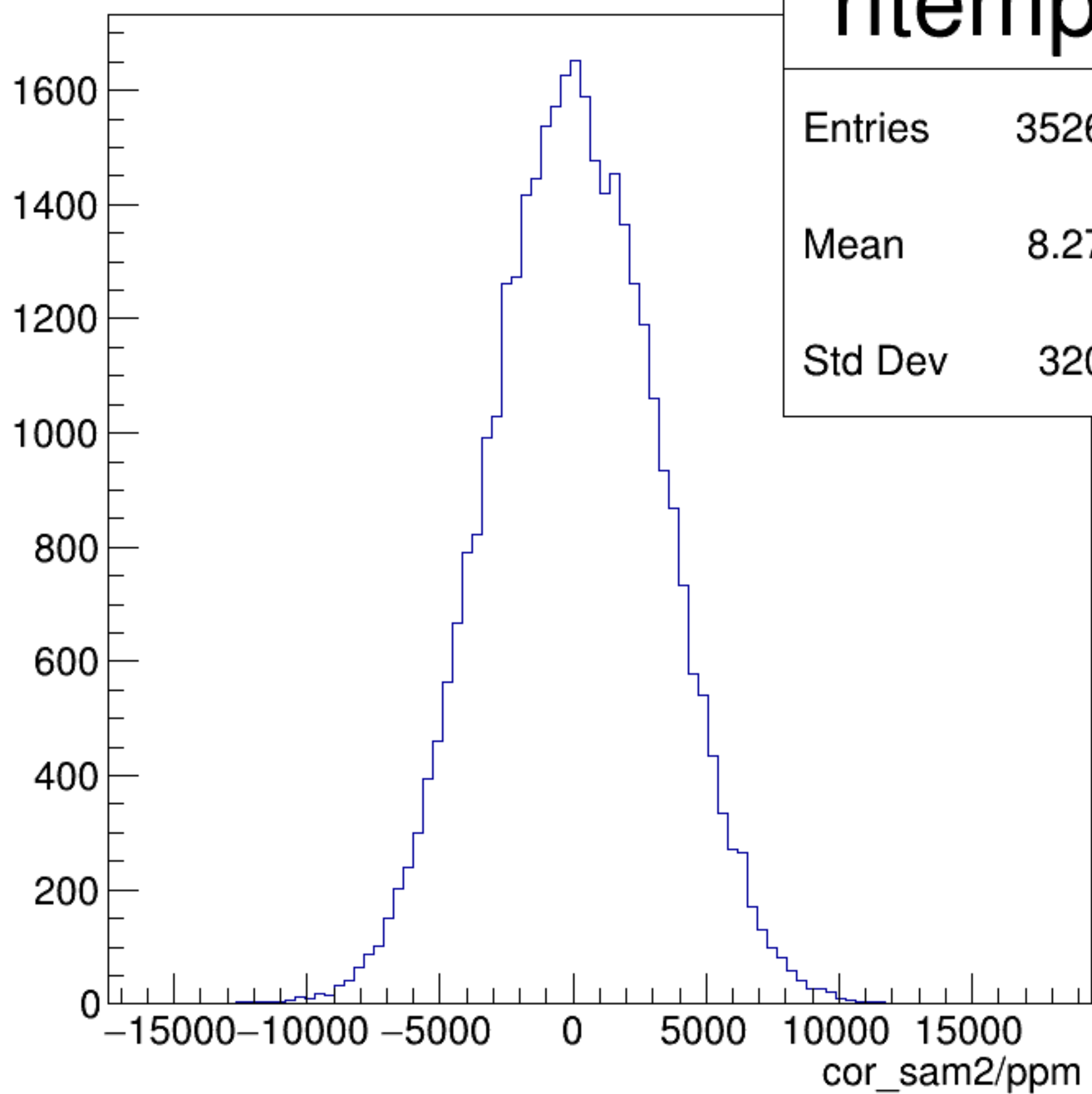
cor_sam2/ppm {ErrorFlag==0}
